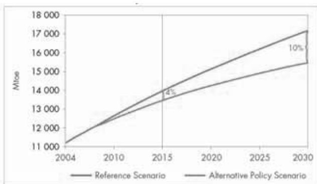
Fig.8. Domanda di energia nello scenario alternativo IEA
