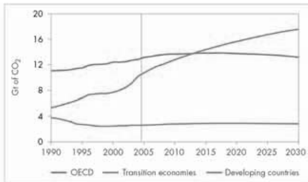
Fig.9. Emissioni di CO 2 nello scenario alternativo IEA
