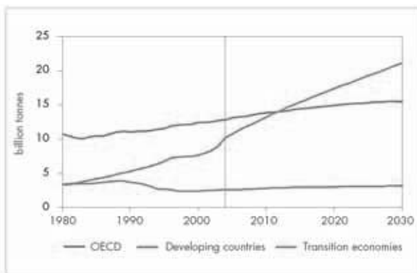
Fig.5. Emissioni di CO 2 legate all'energia per area
