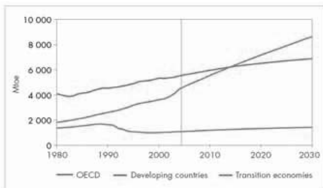
Fig.4. Domanda di energia per area.
