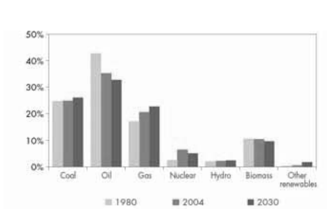
Fig. 3. Quota dei combustibili sulla domanda mondiale
