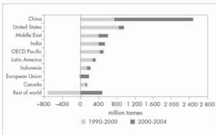
Fig.6. Variazioni nelle emissioni di CO2 per area
